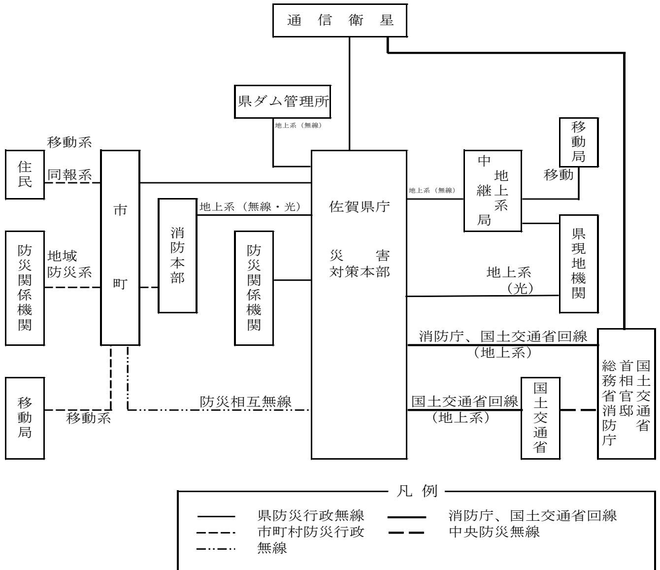
【 通 信 系 統 図 】
