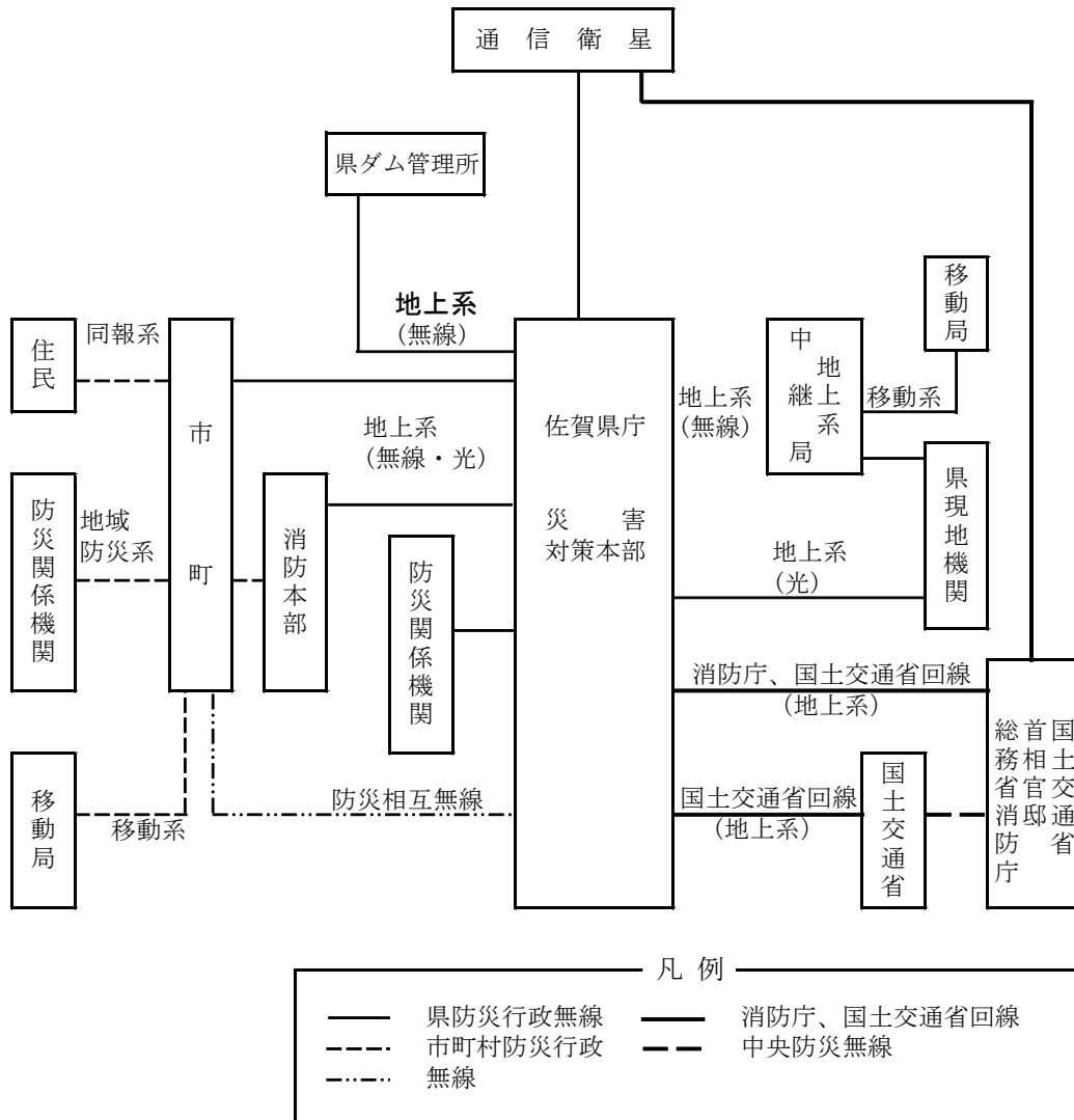
【 通信系統図 】
