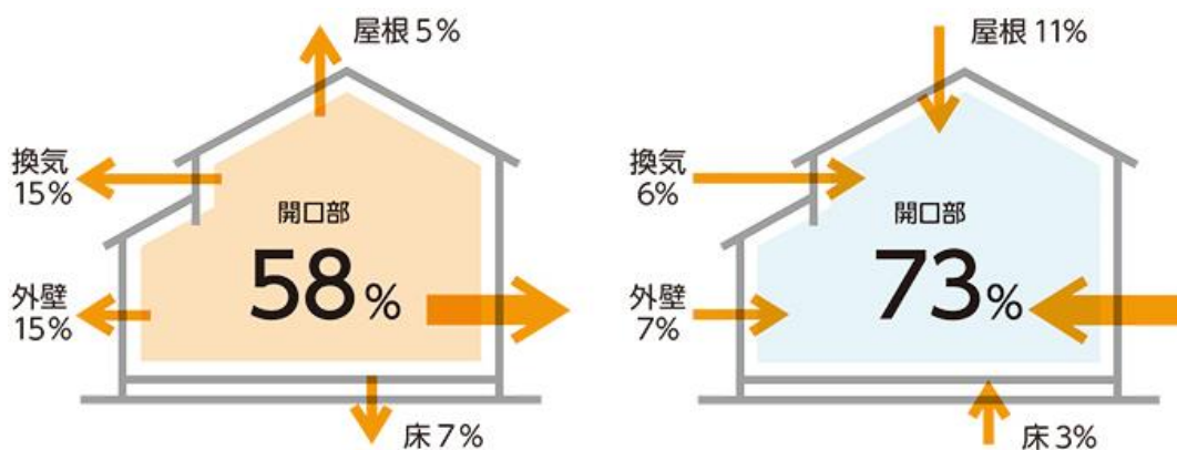
冬の暖房時(左)、夏の冷房時の部屋の熱の出入り
