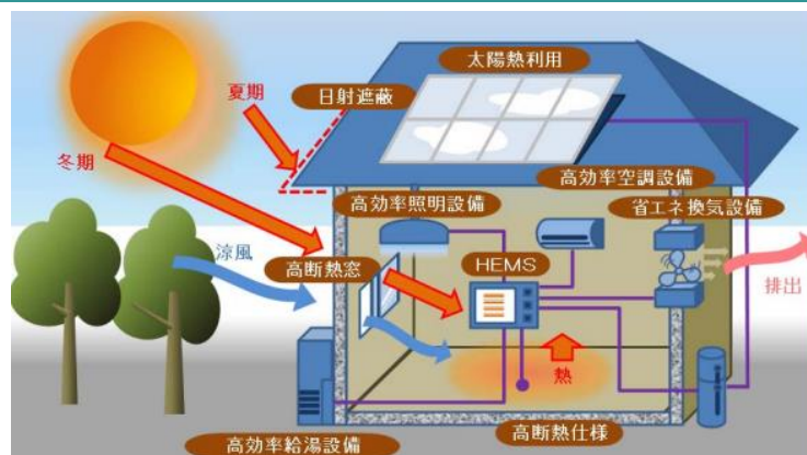
ZEH 住宅の概観
