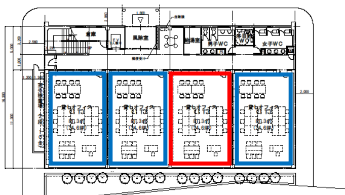
1階平面図
